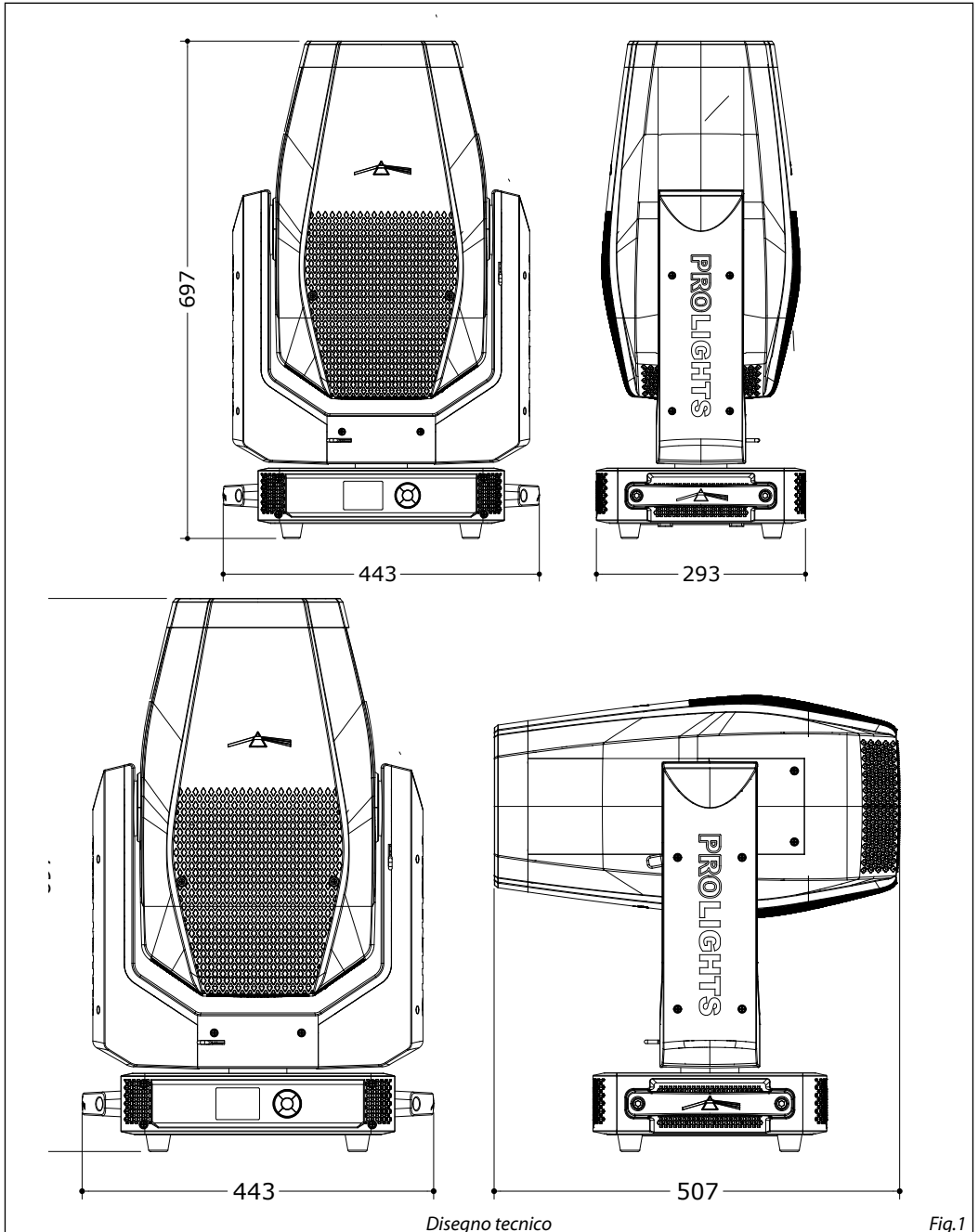
Disegno tecnico
